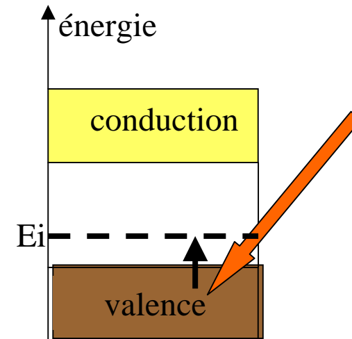
Photoconduction extrinsèque
